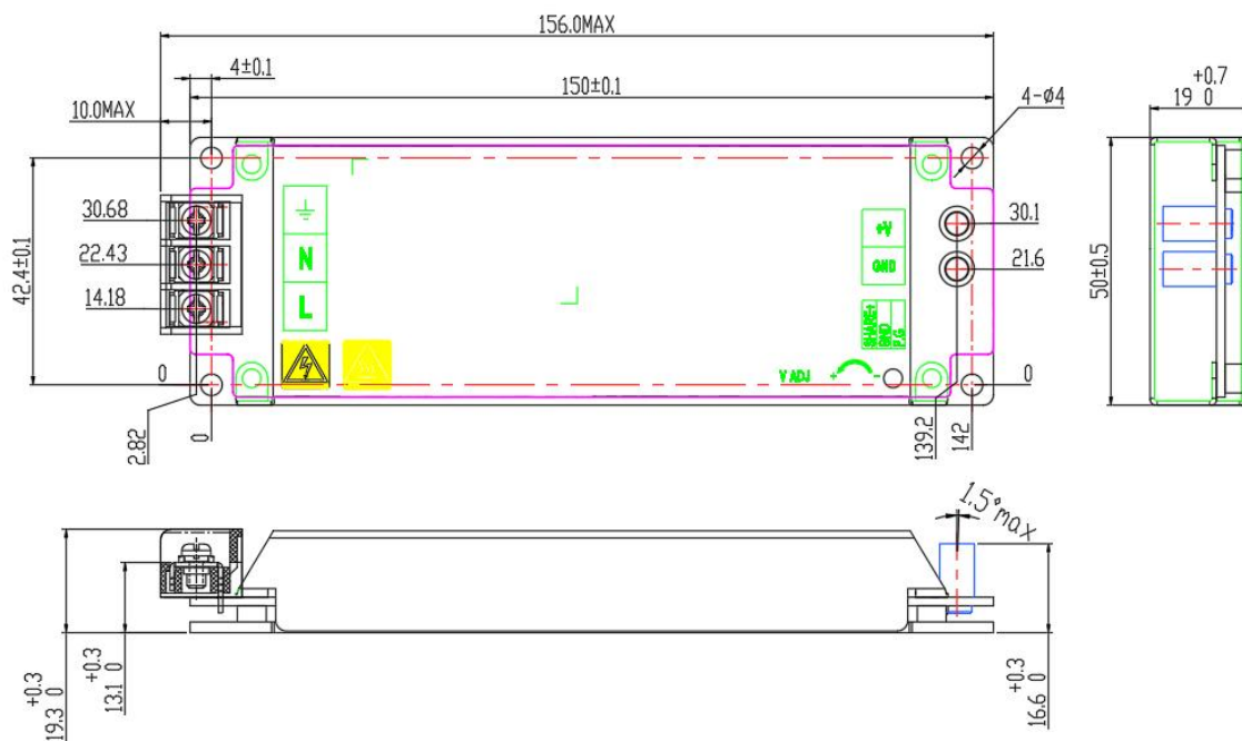
外形尺寸及安装孔——端子坐标图
